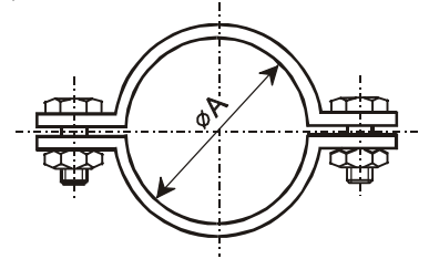
OBJÍMKA OBJ. ČÍS. 3 001 000
