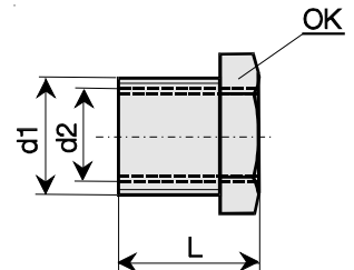
REDUKCE TYP 2518 OBJ. ČÍS. 3 004 177
