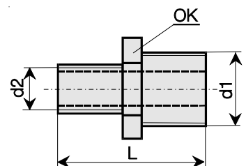
REDUKCE TYP 4116 OBJ. ČÍS. 3 004 209
