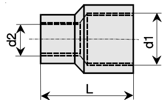
REDUKCE TYP 3512 OBJ. ČÍS. 3 004 197
